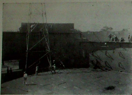
Vista interior de un tanque de 80.000 barriles.
