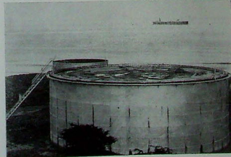
Los primeros tanques de madera para petróleo.
