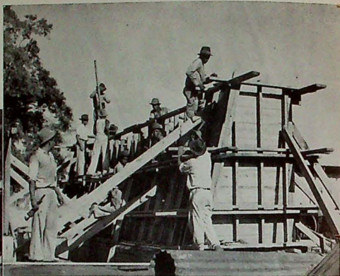
Colocando armazón para estribos del puente.
