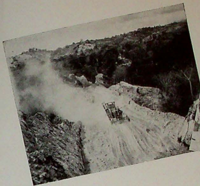
Cuchilla trabajando en corte en el Cerro del Diablo.
