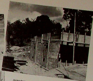
Armadura colocada después de echar pared de concreto del tanque de abastecimiento.
