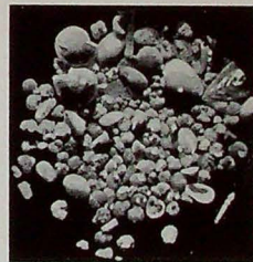
Otras especies de foraminíferos, 25 veces aumentadas.
