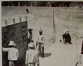
Colocando armadura y barras de refuerzo para pared divisora en el centro del tanque de abastecimiento.
