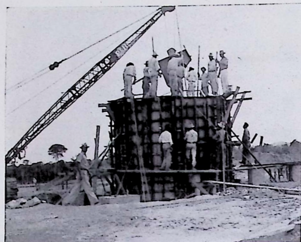
Construcción de una de las torres para las labores industriales de la refinería.
