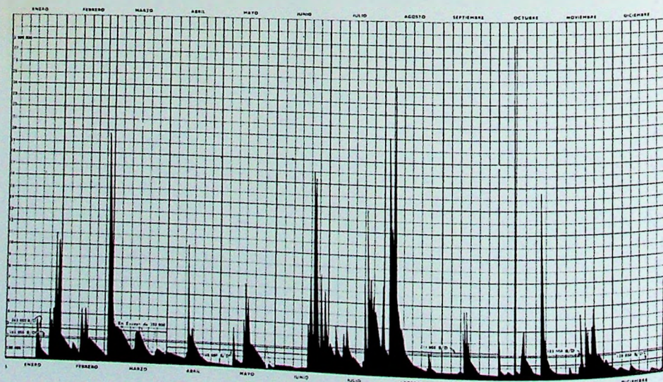
GRAFICO DEL GASTO PARA EL AÑO 1948 DEL RIO SIBURUA MEDIDA DEL VERTEDERO No. 1
