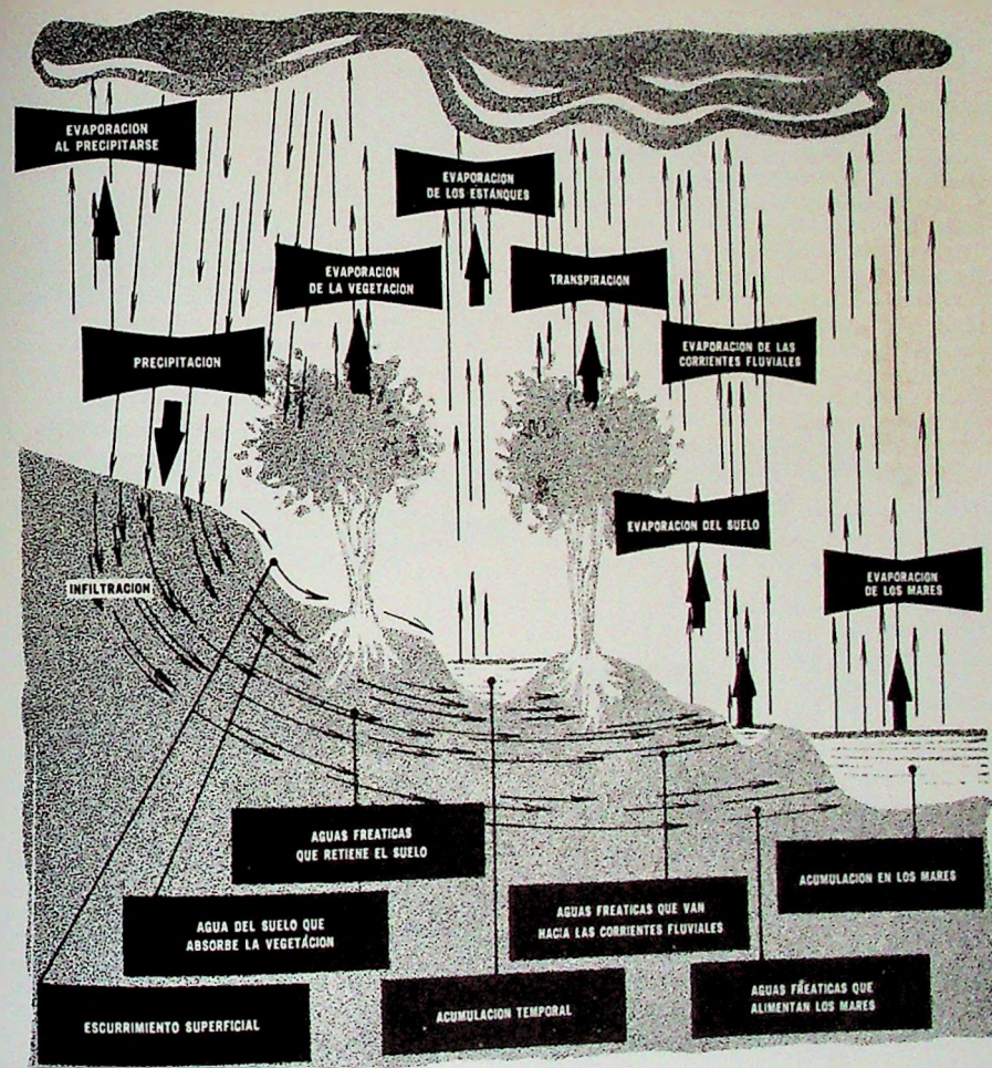
Fig. 1. — El ciclo hidrológico.
